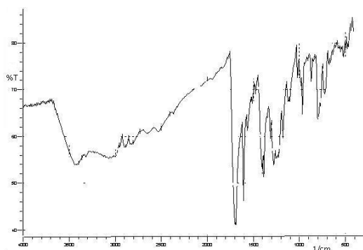
Fig. 2 IR spectrum of TCPP
