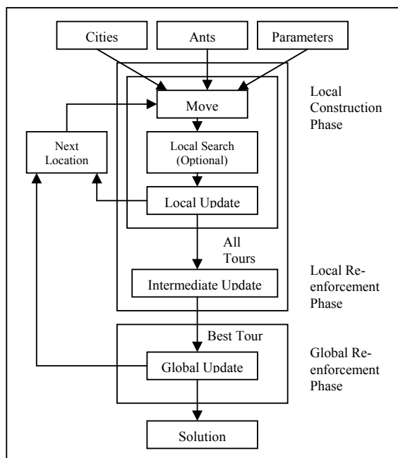
Fig. 3 DACS3 Diagram
