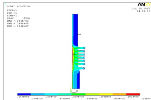
Fig. 7 Von-Mises Stress
