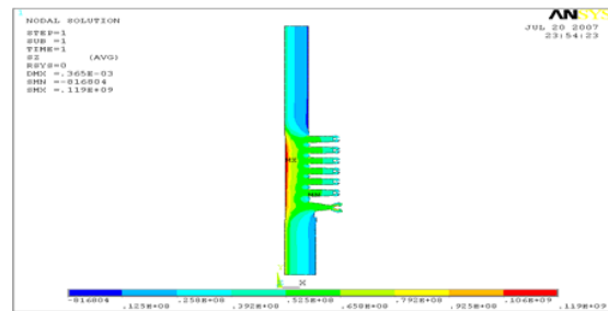
Fig. 10 Max Hoop Stress
