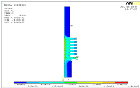
Fig. 11 Von-Mises Stress
