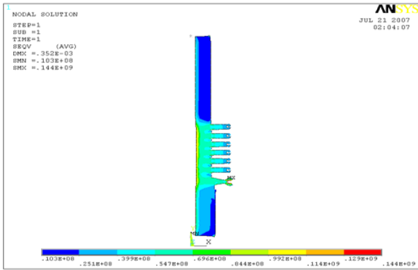
Fig. 13 Von-Mises Stress
