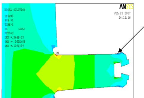
Fig. 5 Max Radial Stress
