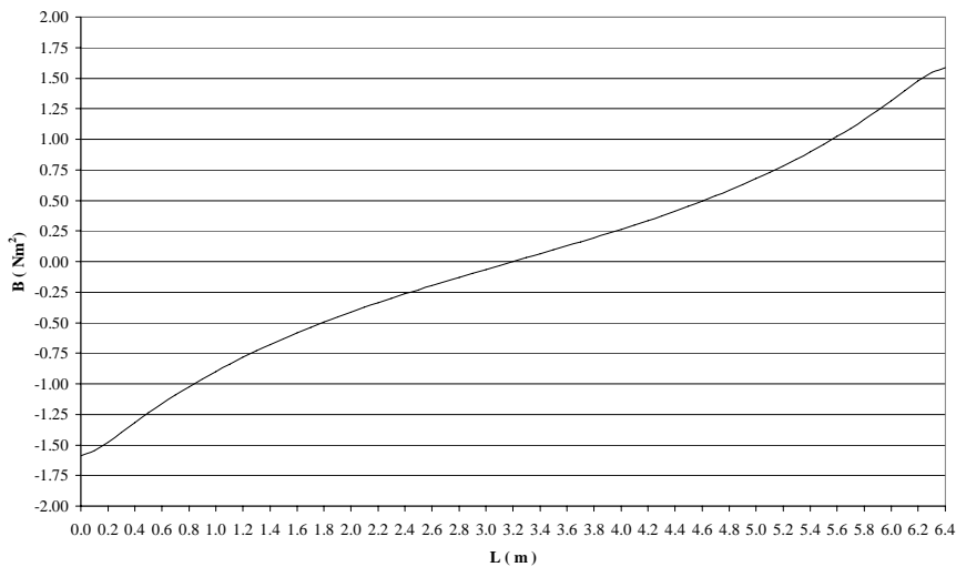
Fig. 6 Bimoment longitudinal distribution
