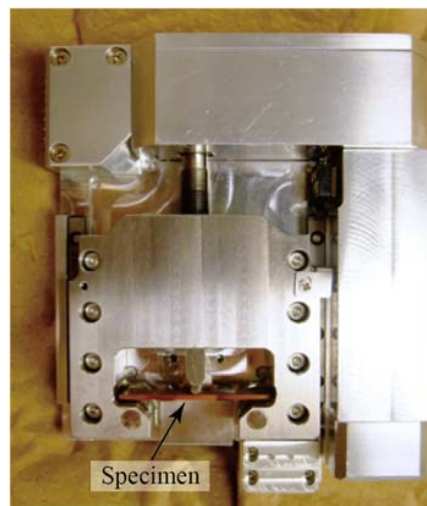
Fig. 2 Bending apparatus
