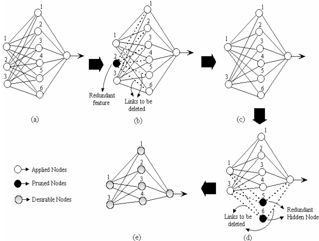
Fig. 6 Optimization of neural network (a) input nodes (d) hidden nodes
